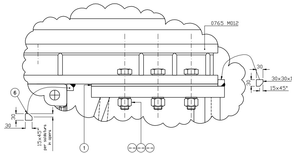
PARTICOLARE X Scala 1:5
